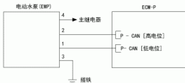
〔电路图〕
